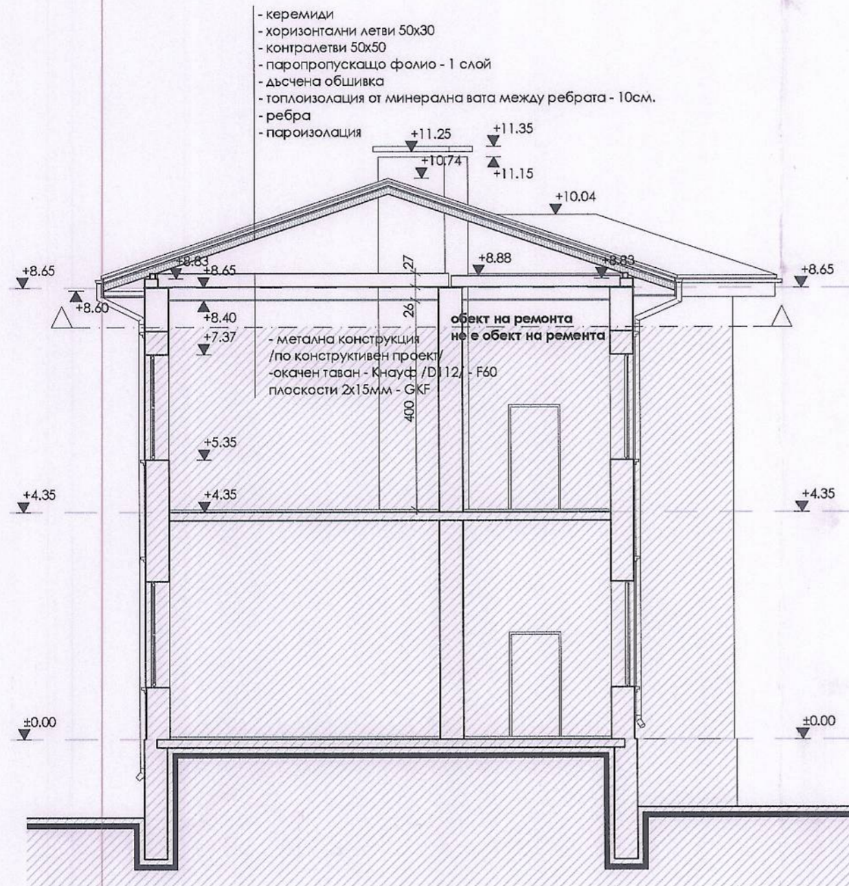
Разрез А-А
